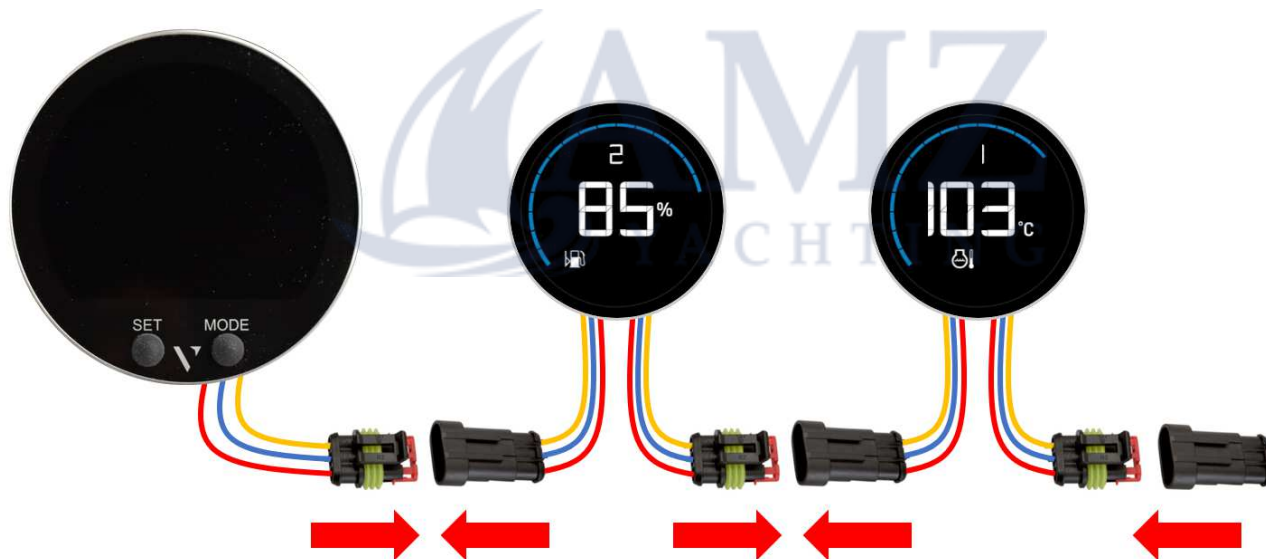
Collegamento EasyLink con il master VMH 35 e due satelliti VMH 14 in cascata
